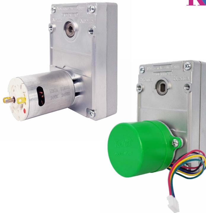
VERSIONE DC 24V - 24V DC MODEL
